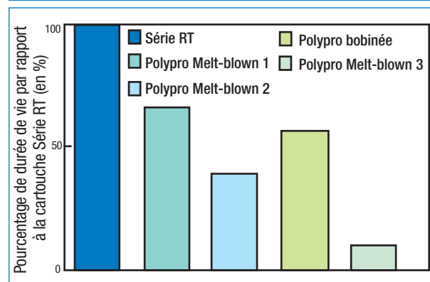
Schéma 3 - Comparaison de la durée de vie de différentes cartouches filtrantes montrant une efficacité équivalente
