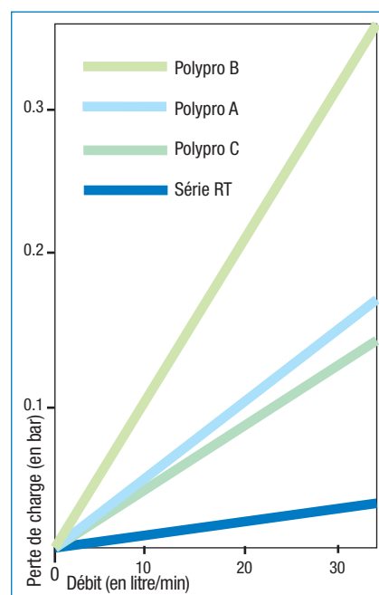
Schéma 4 Débit en fonction de la perte de charge
