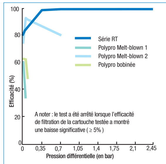
Schéma 1 - Efficacité comparée de plusieurs cartouches filtrantes de seuil équivalent
